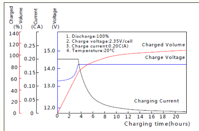
Charakterystyka ładowania
