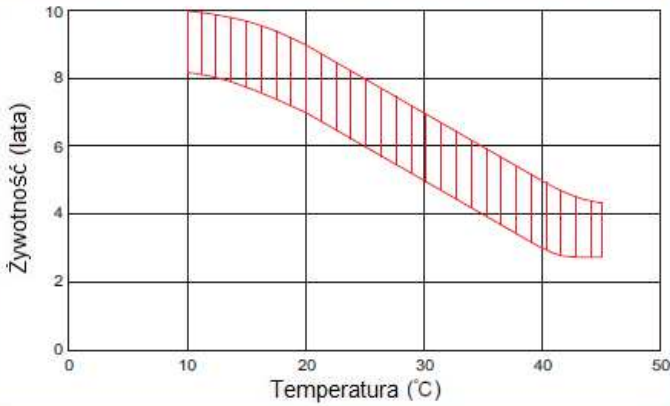
Projektowana żywotność w zależności od temp.
