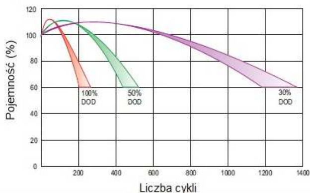
Żywotność cykliczna w zal. od głębokości rozładowania
