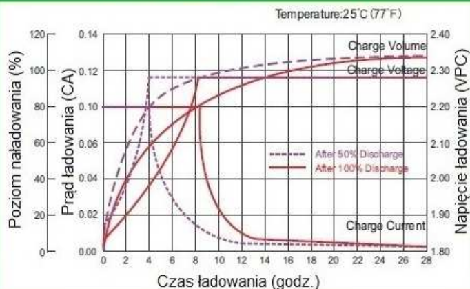
Charakterystyka rozładowania
