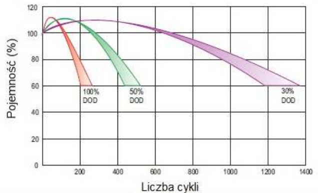
Żywotność cykliczna w zał. od głębokości rozładowania
