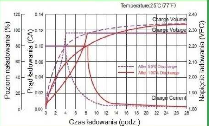
Charakterystyka rozładowania
