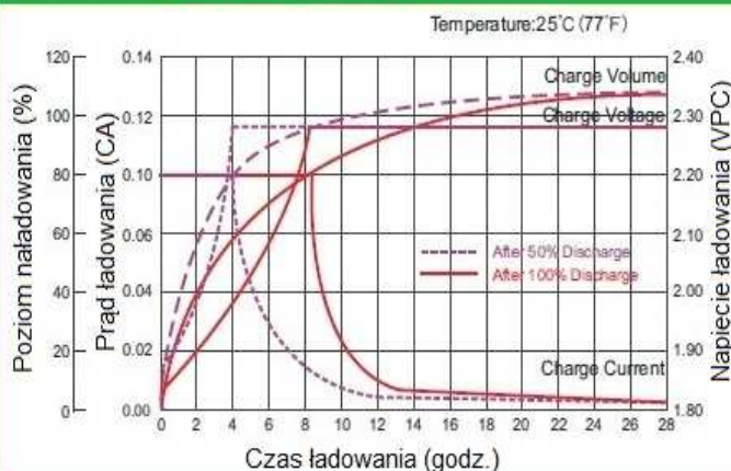
Charakterystyka rozładowania
